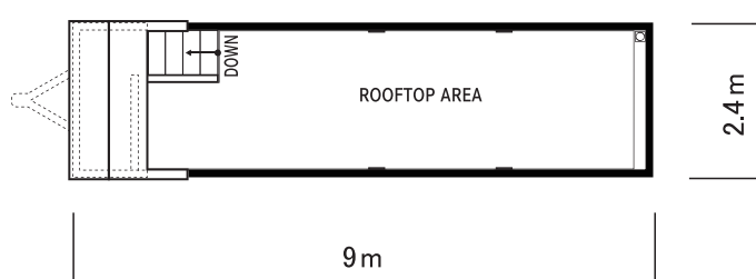
【平面図・屋上】
