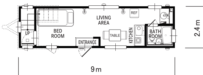
【平面図・室内】
